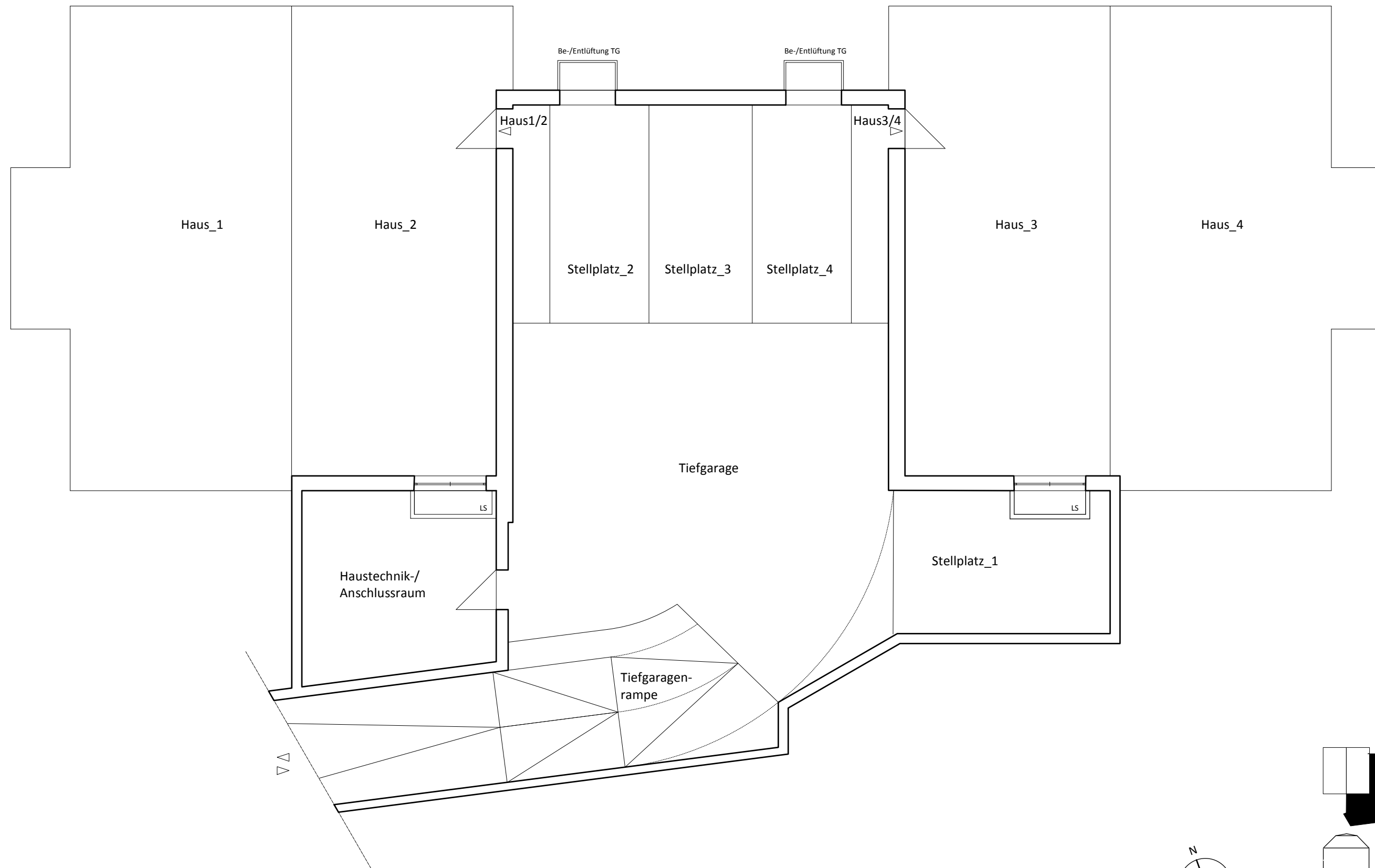
Tiefgarage Übersicht
